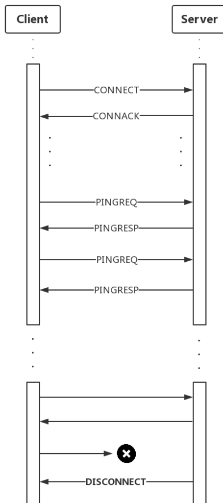
图 2 MQTT 心跳机制
